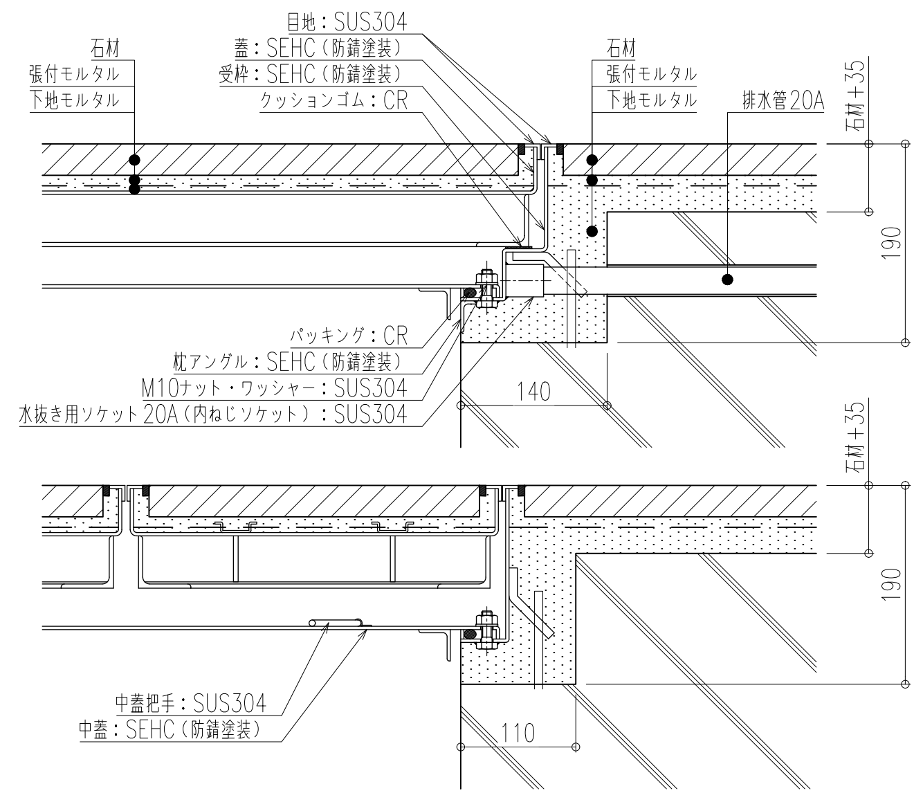
施工参考拡大図
