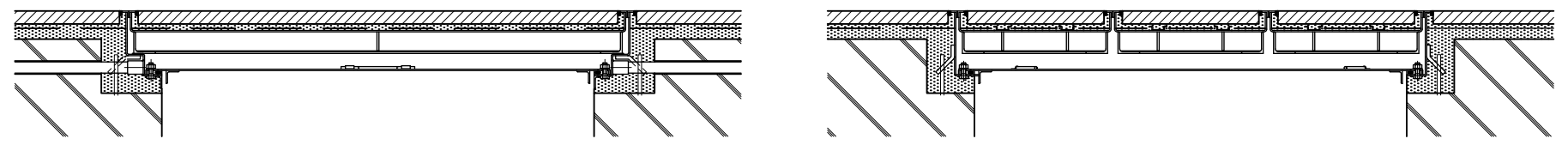
施工参考図
